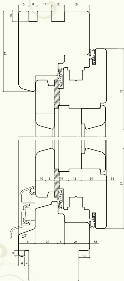
Przekrój okna w systemie DJ68
