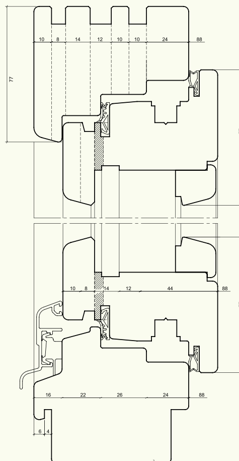
Przekrój okna w systemie DJ88
