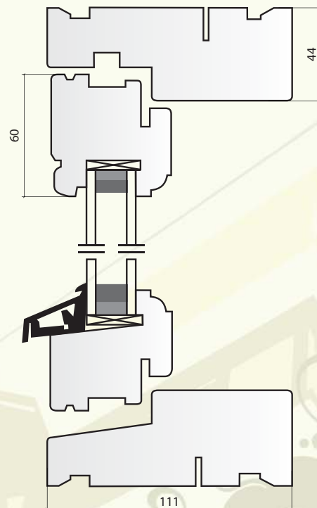
Przekrój pionowy okna o profilu "MILJO". Okno otwierane na zewnątrz.
